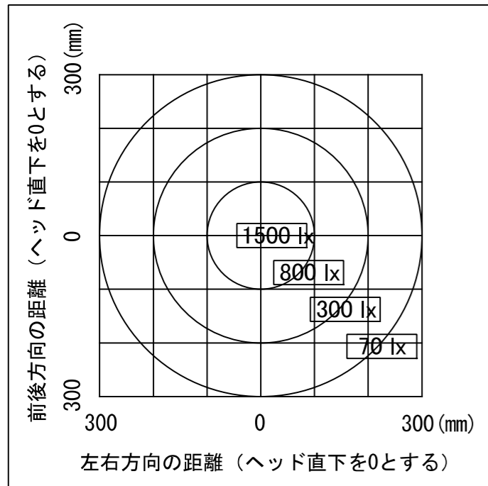
△ 照度分布図
